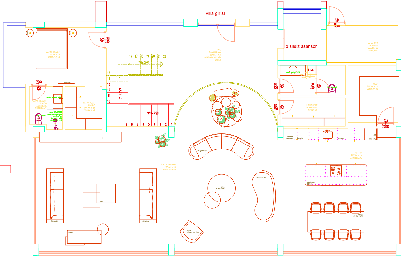
BODRUM KAT PLANI ÖLÇEK: 1/50 GENEL m 2 = 229,65m 2
