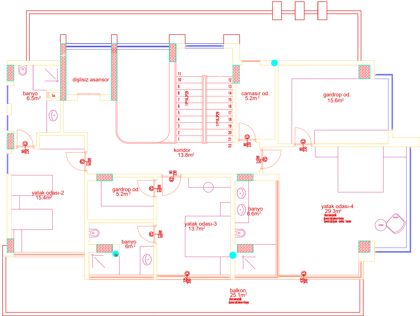
ZEMİN KAT PLANI ÖLÇEK:1/50 GENEL m 2 =152.98m 2
