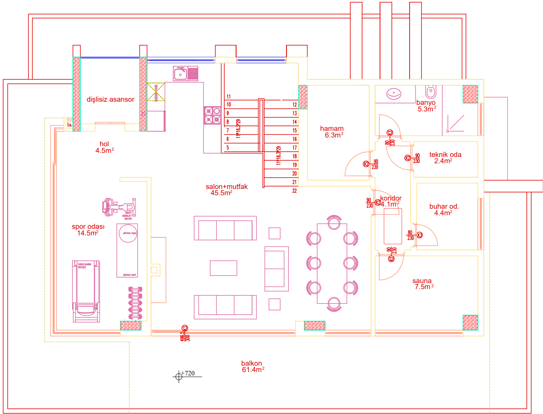
I. KAT PLANI ÖLÇEK:1/50 GENEL m 2 =165.43m 2
