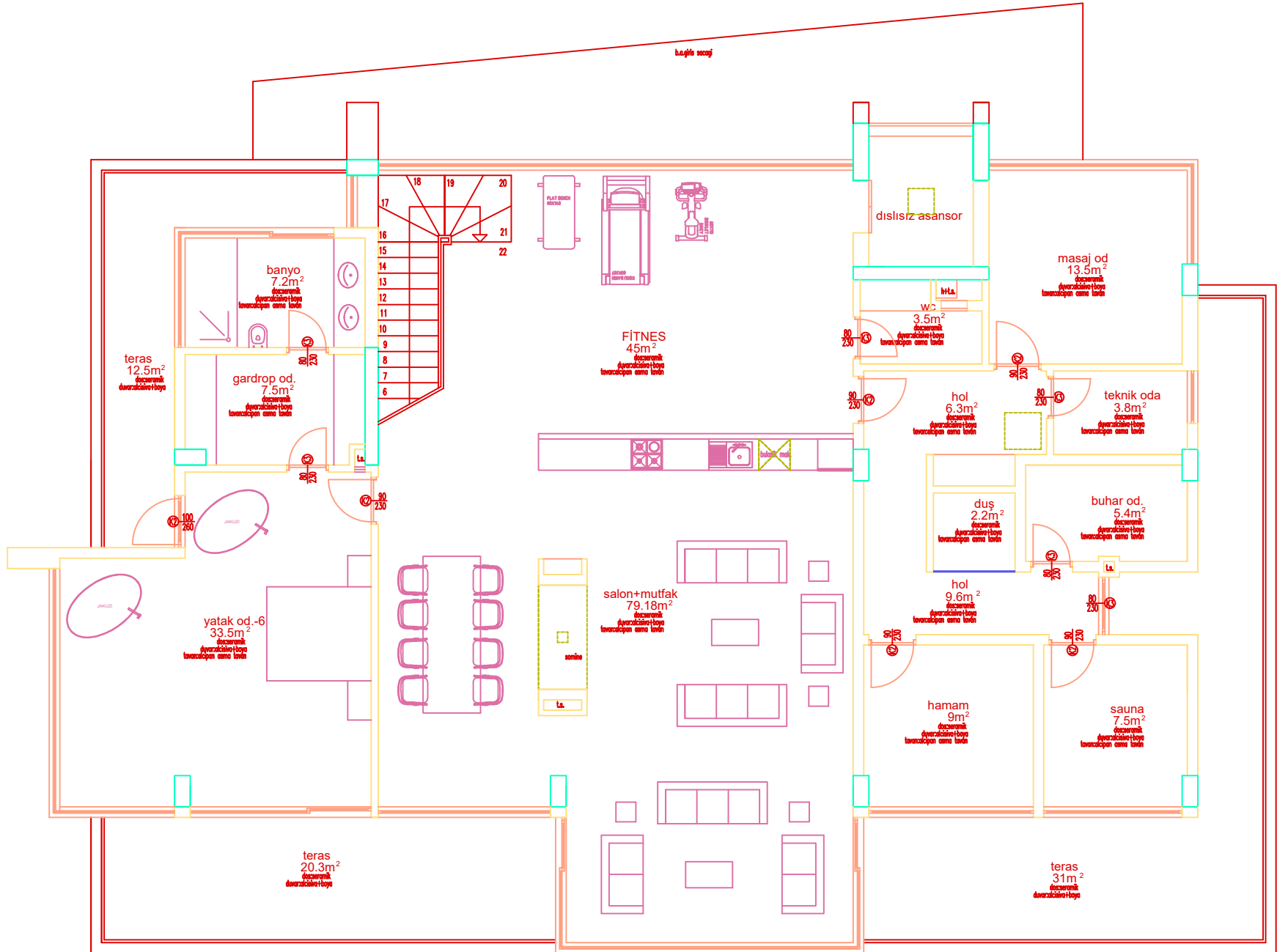
1. KAT PLANI ÖLÇEK:1/50 GENEL m 2 =273.18m 2
